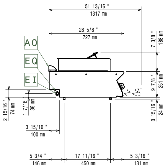
Oldalnézet
