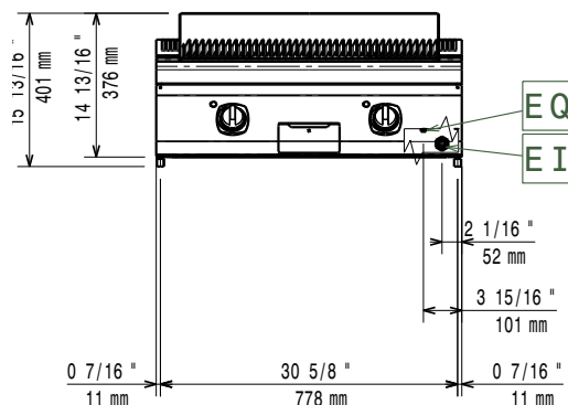
Előlnézet
